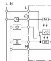
— Schaltbild UTE 1033
