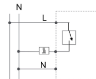
Schaltbild UTE 2100
