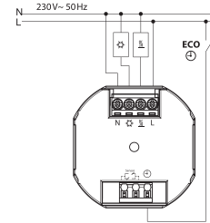
Schaltbild UTE 4100-Rw
